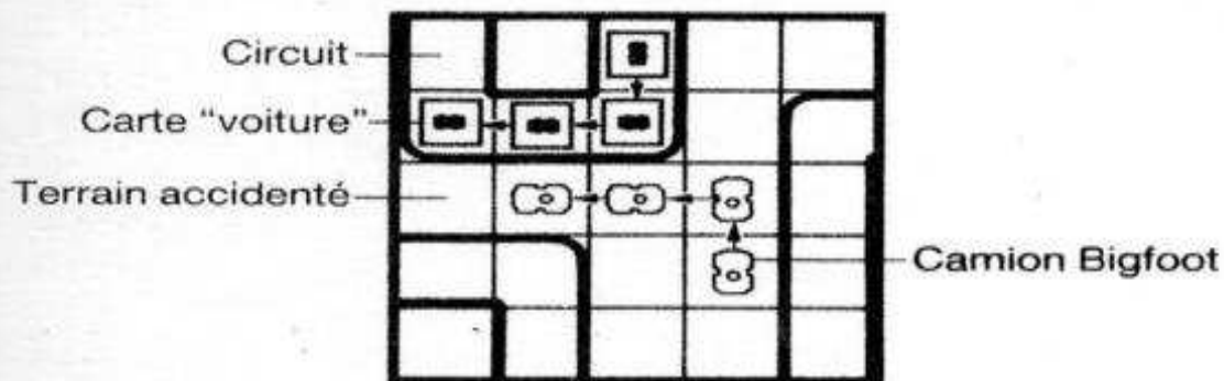
Fig.2 Exemple de déplacement si chacun des deux dés indique 3.
